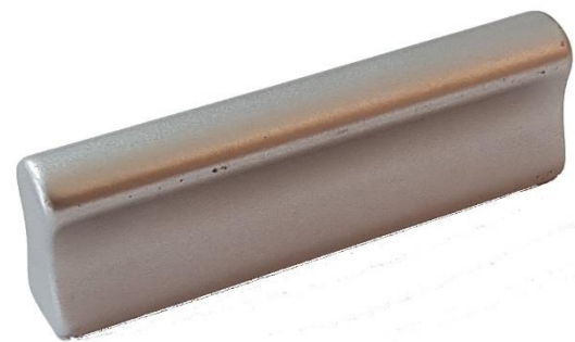
Ref. 788 Tirador ABS 75 x 19 x 10 mm 32 mm entre taladros
