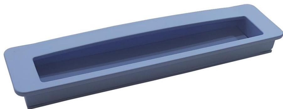
Ref. 753 Tirador ABS 180 x 45 mm encastrable 12 mm 160 mm entre taladros
