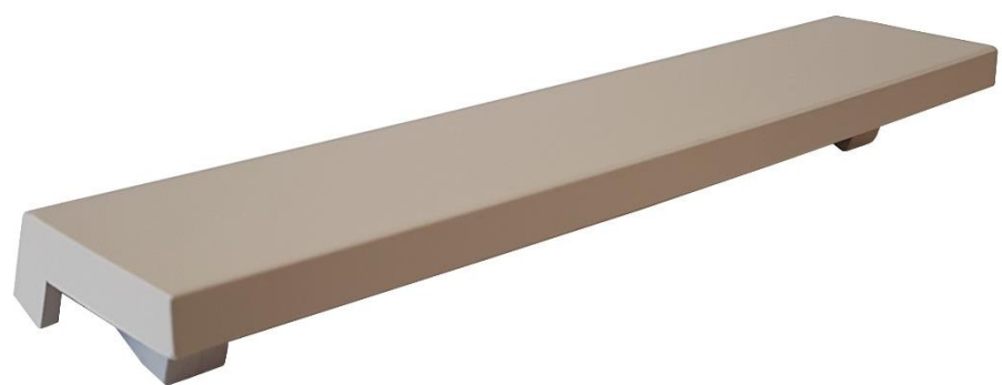
Ref. 525 Tirador ABS 200 x 29 x 40 mm 160 mm entre taladros
