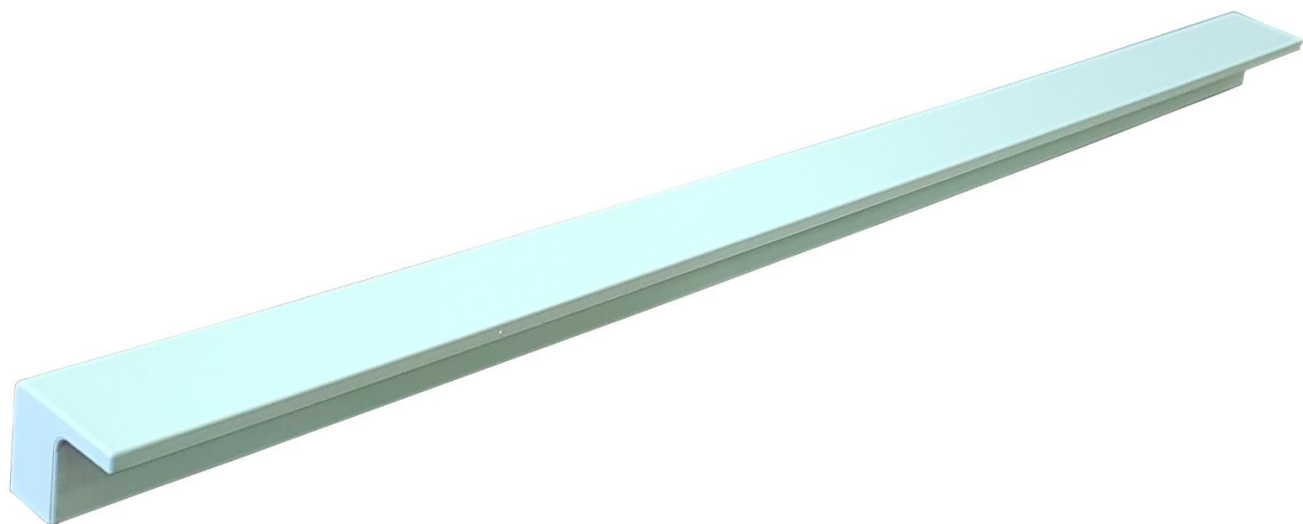
Ref. 601 Tirador ABS 410 x 20 x 25 mm 320-128 mm entre taladros
