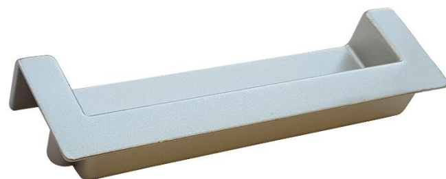
Ref. 624 Tirador ZAMAK 110 x 32 encastrable 14 mm 96 mm entre taladros
