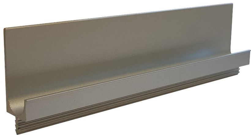
Ref. 732 Tirador ALUMINIO 35 x 16 mm, para tablero de 16 y 19 mm Cortado y mecanizado a medida
