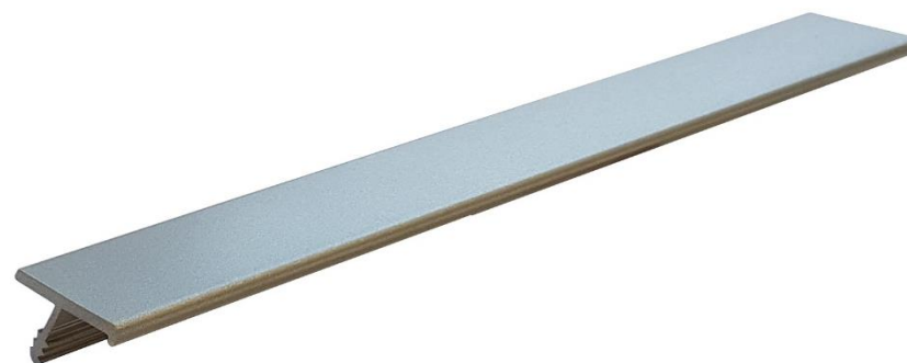
Ref. 731 Tirador ALUMINIO ángulo 50 grados, para tablero de 16 mm Cortado y mecanizado a medida
