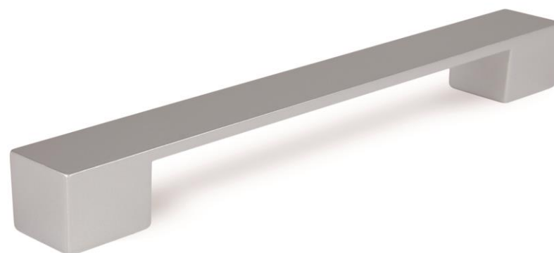
Ref. 780 Tirador ZAMAK 27 x 25 mm 248 x 224 mm entre taladros 200 x 160 mm entre taladros 162 x 128 mm entre taladros
